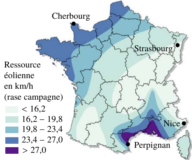
Figure 3 – La ressources éolienne en France.
