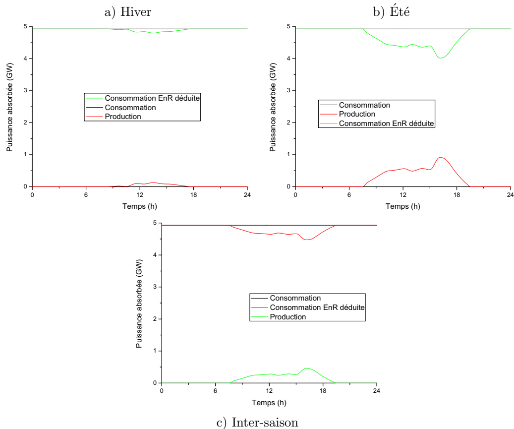
Figure 4.19 – Courbes de charge du modèle I6
