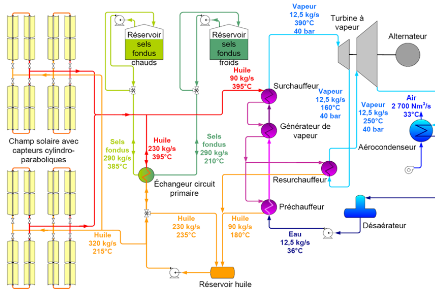
Figure 1.3 – Une centrale solaire thermodynamique avec stockage.
