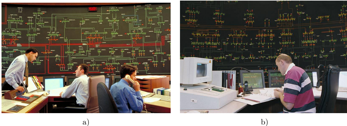
Figure 1.19 – Centres de dispatching énergétique français. a) St Quentin en Yvelines - b) Lyon
