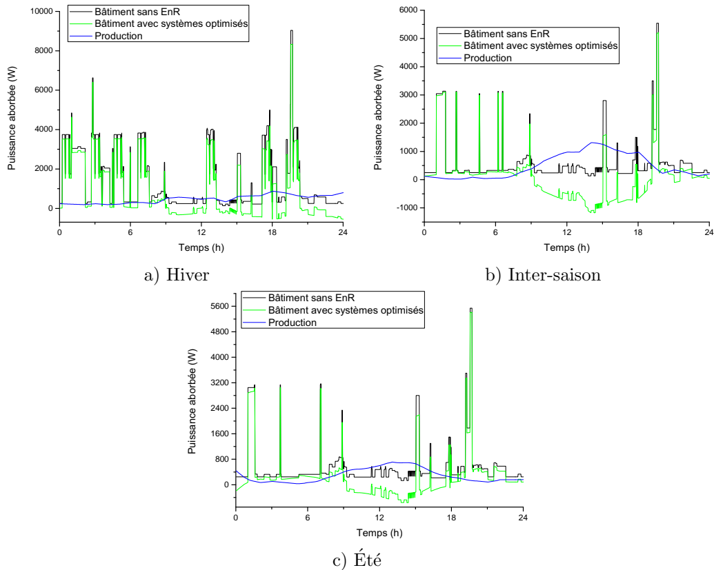
Figure 4.14 – Courbes de charge du modèle n°10 avec minimisation de l'IER
