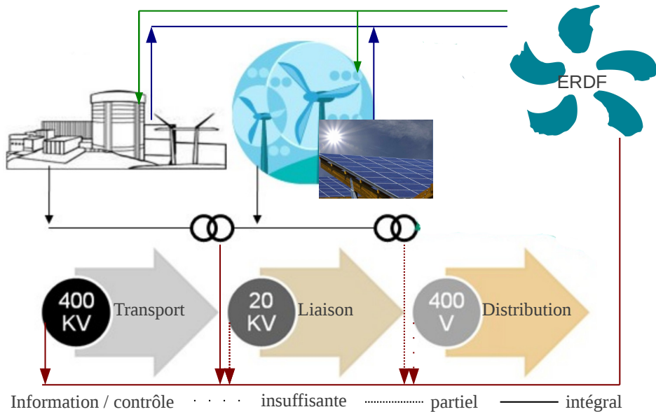
Figure 1.15 – Schéma d'un réseau électrique
