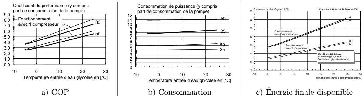
Figure 3.57 – Courbes caractéristiques du fonctionnement d'une pompe à chaleur eau/eau utilisée pour chauffer un bâtiment mal isolé de 180 \text{ m}^2
