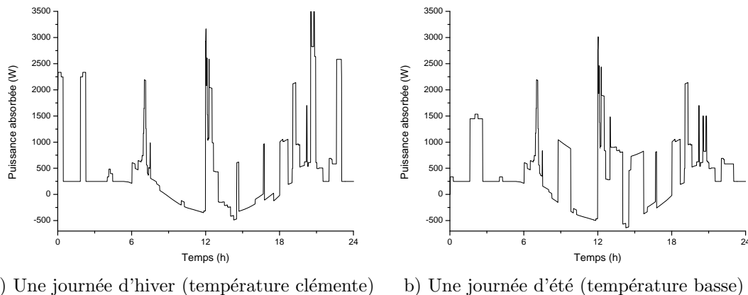
Figure 4.3 – Courbes de charge du modèle n°1
